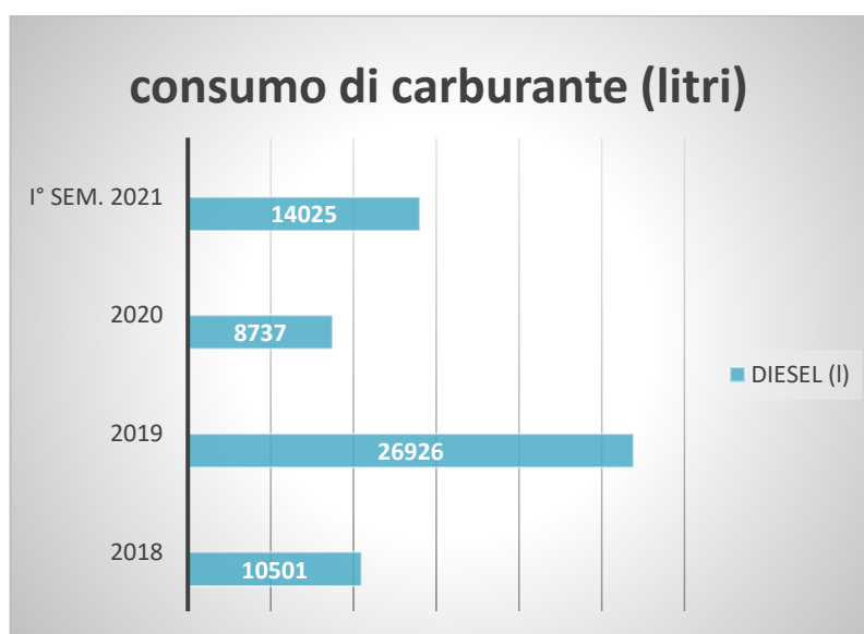
Fig.5 Andamento consumi carburante
